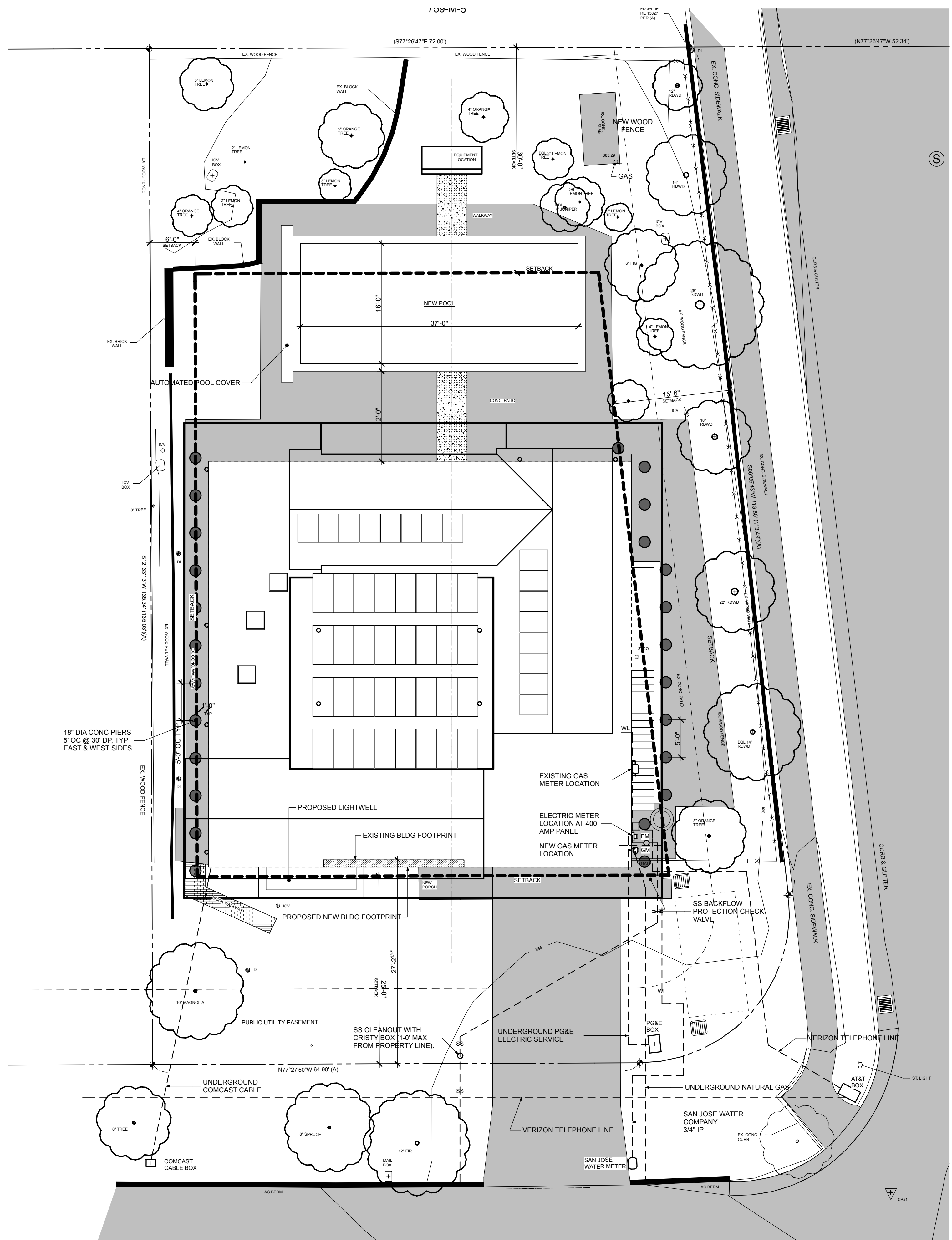
1 Utilities Plan Scale: 1/8" = 1'-0"
